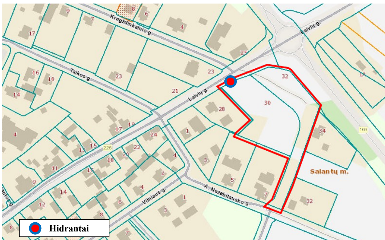
3.7.1 pav. Hidrantų išsidėstymas planuojamos teritorijos gretimybėse (šaltinis: UAB „Kretingos vandenys“)
