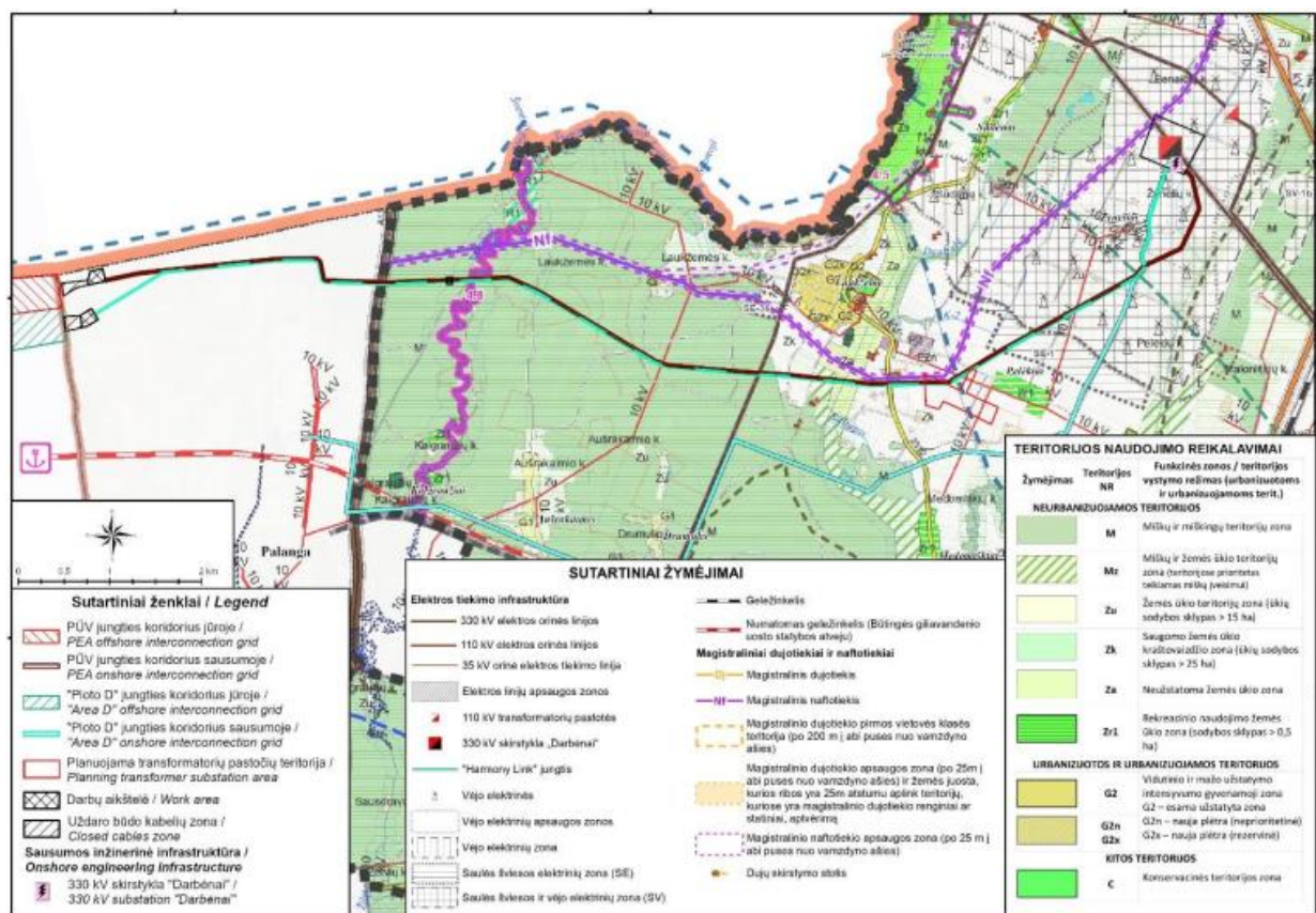
5.12.1. pav Jungčių trasų išsidėstymas Kretingos rajono teritorijoje The route of the connections within the territory of Kretinga district
