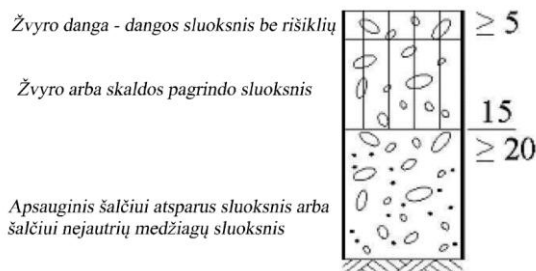
5.14.1 pav. Žvyro kelio atstatymo schema.
