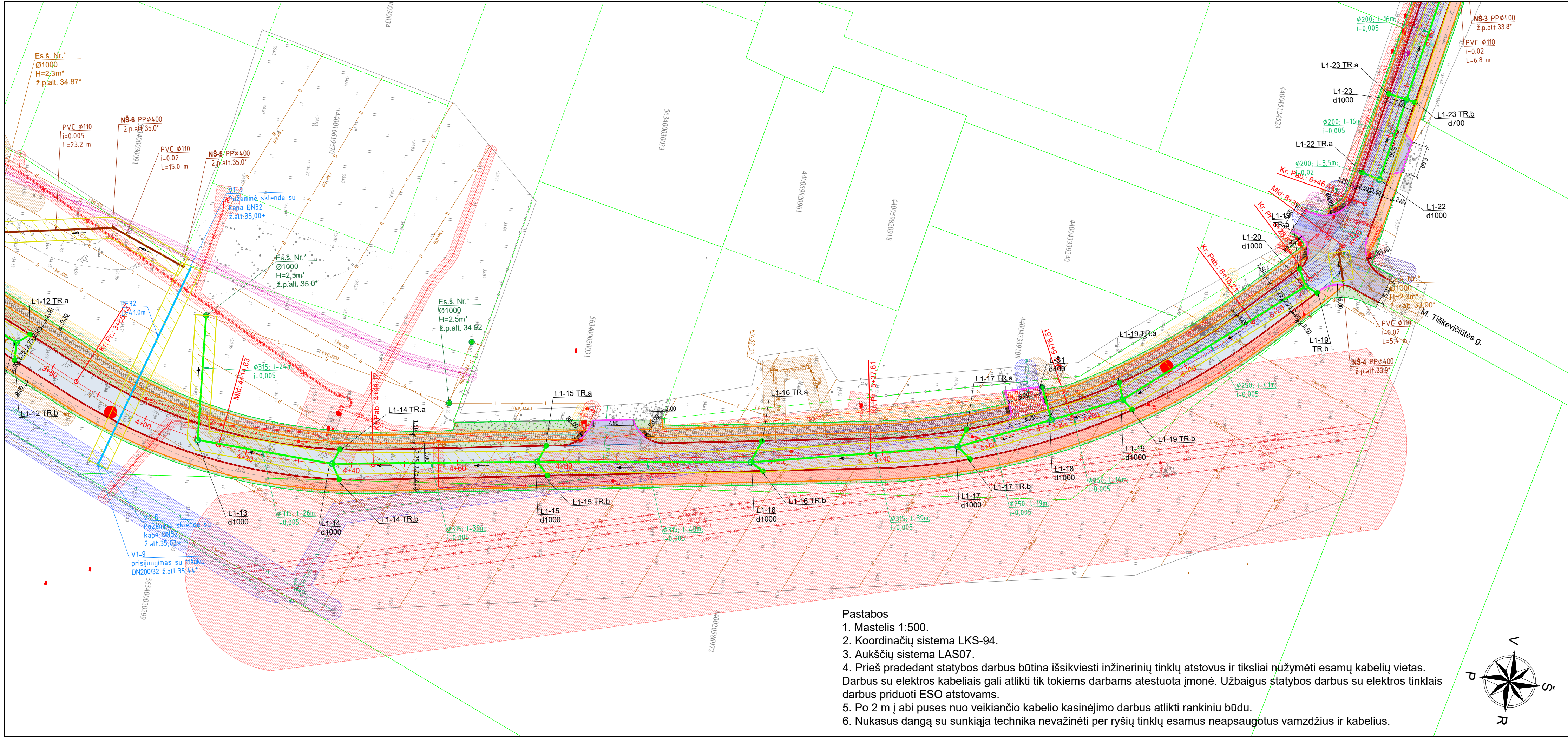
LAPŲ IŠDĖSTYMO SCHEMA
