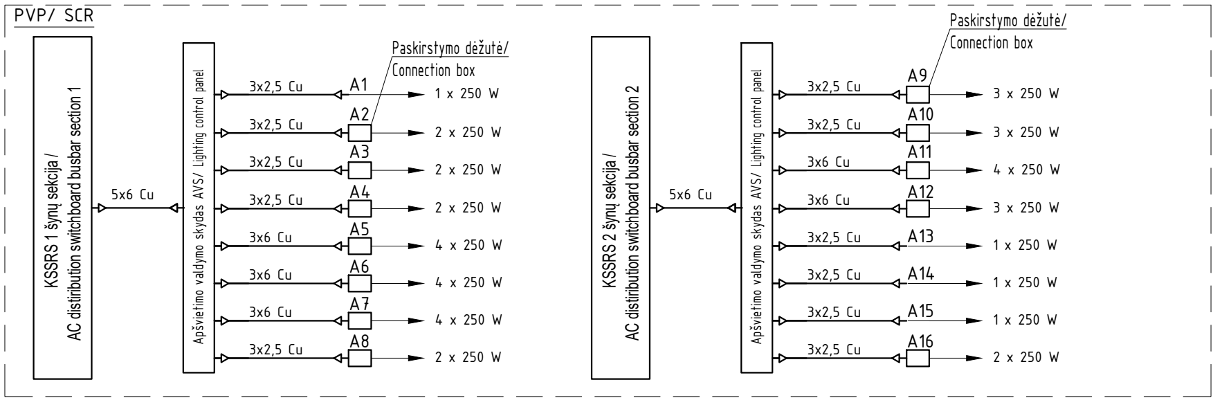
Pastotės teritorijos apšvietimo tinklo schema/ Substation area lighting network diagram
