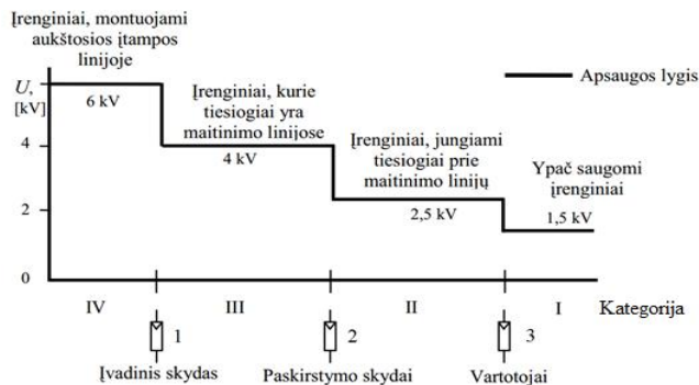
4 pav. Ribotuvių klasės pagal saugomą objektą /
