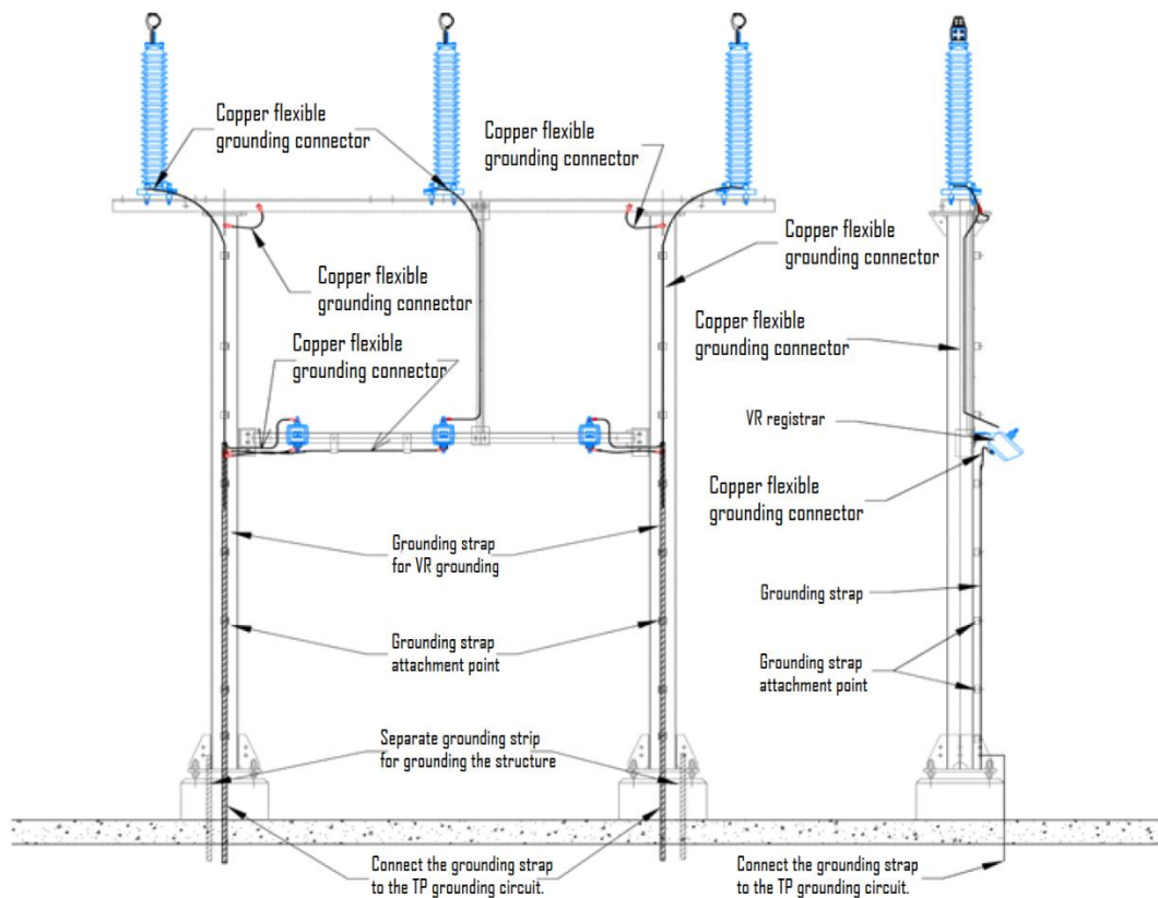
7b pav./ picture: viršįtampių ribotuvas pastatytas ant laikinės konstrukcijos su dviem kolonom./ Surge arrester mounted on supporting construction with two poles
