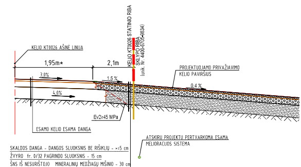
SKALDOS DANGOS NUVAŽOS IŠILGINIS PJŪVIS 1-1
