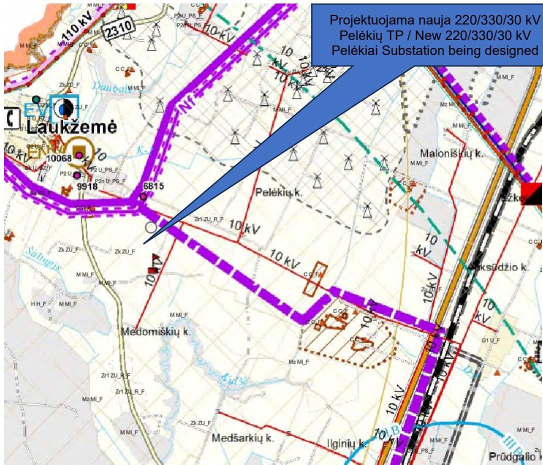
3 pav. Planuojamo statyti statinio schema inžinerinės infrastruktūros vystymo plano brėžinio kontekste / Fig. 3. Schematic diagram of the planned structure within the context of the engineering infrastructure development plan drawing
